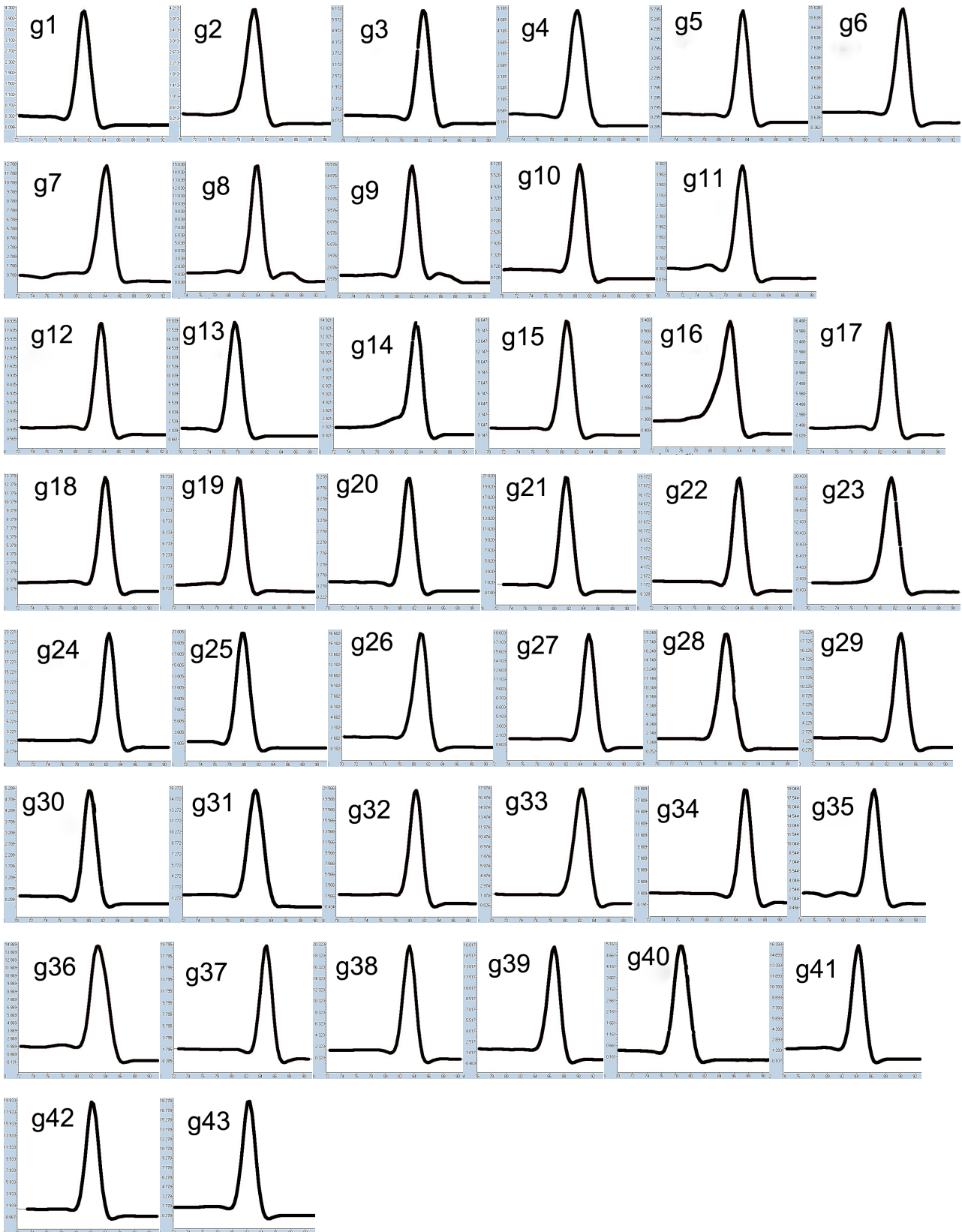
图3 候选内参基因 PCR 产物的溶解曲线
